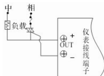
761□ 771□ 接线图例
