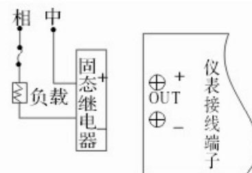
751□ 接线图例
