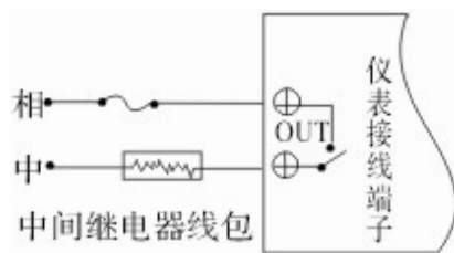
741□ 接线图例
